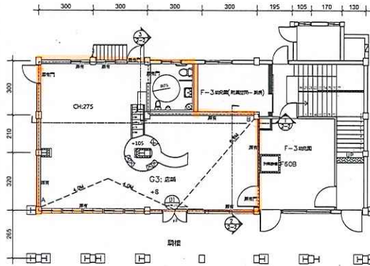
(申請)一層平面圖 S:1/100
