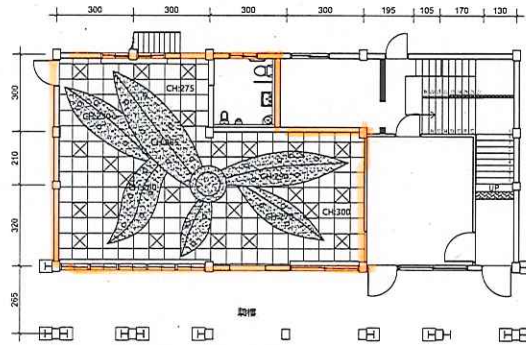
(申請)一層天花板平面圖 S:1/100
