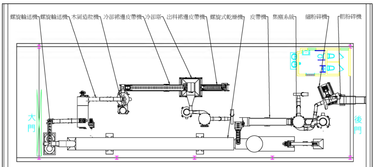
造粒機組配置圖 (圖面僅供參考，依現況為主)
