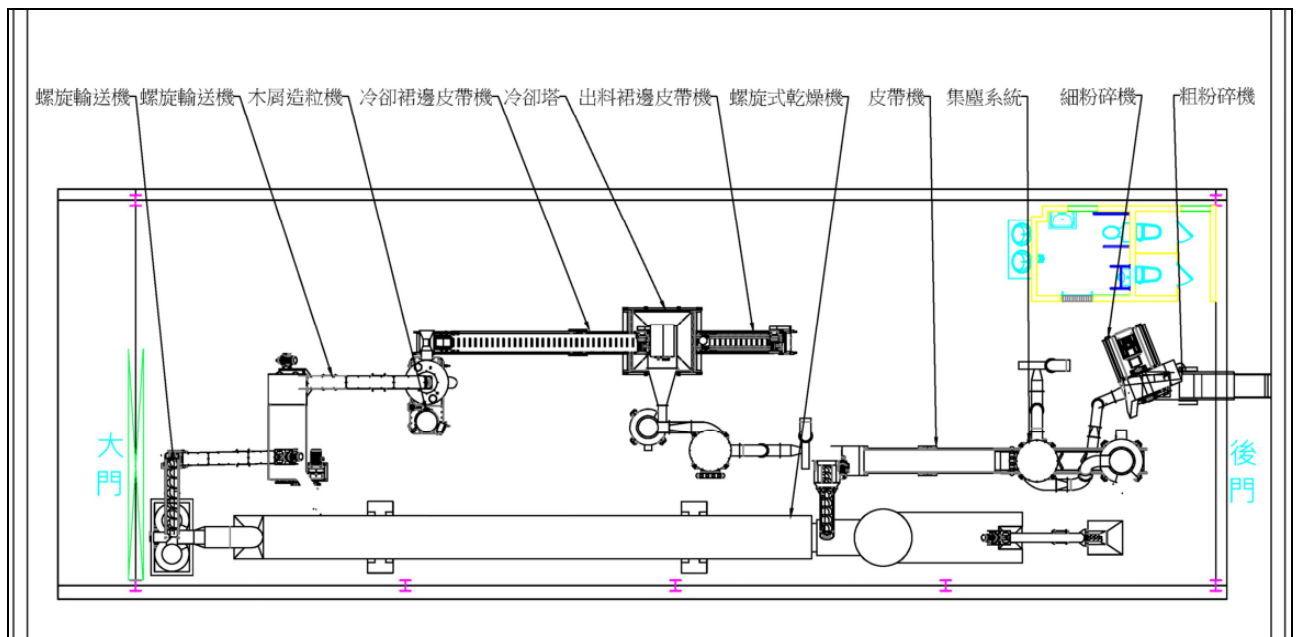
圖 2、造粒機組配置圖（圖面僅供參考，依現況為主）
